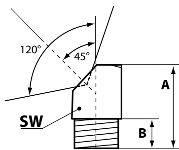
15 707 M 6 x 1-VZ-SK-SW 11 A: 16 B: 5,5
