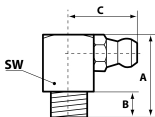
15 207 M 6 x 1-VZ-VK-SW 9 A: 18 B: 5,5 C: 14
