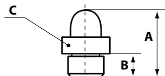
15 309 M 8 x 1-VZ-SK-SW 9 A: 14 B: 5,5
